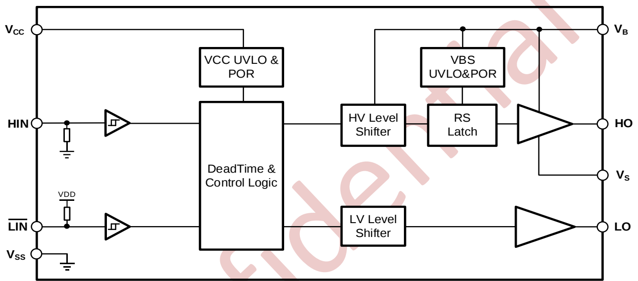
图 10-1 G2025 功能框图
